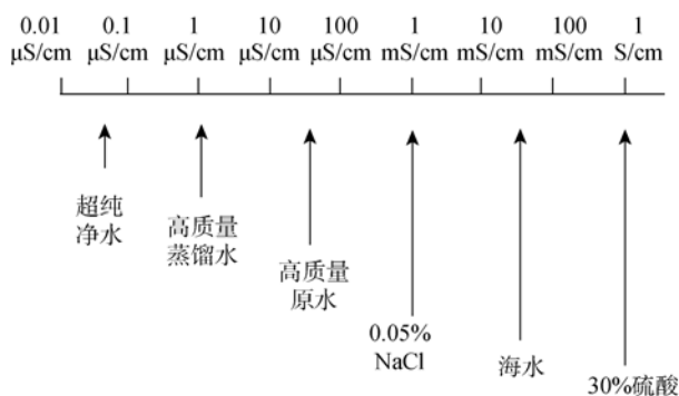
图2 不同溶液(液体)的电导率差异(Rosemount Analytical Inc., 2010)
