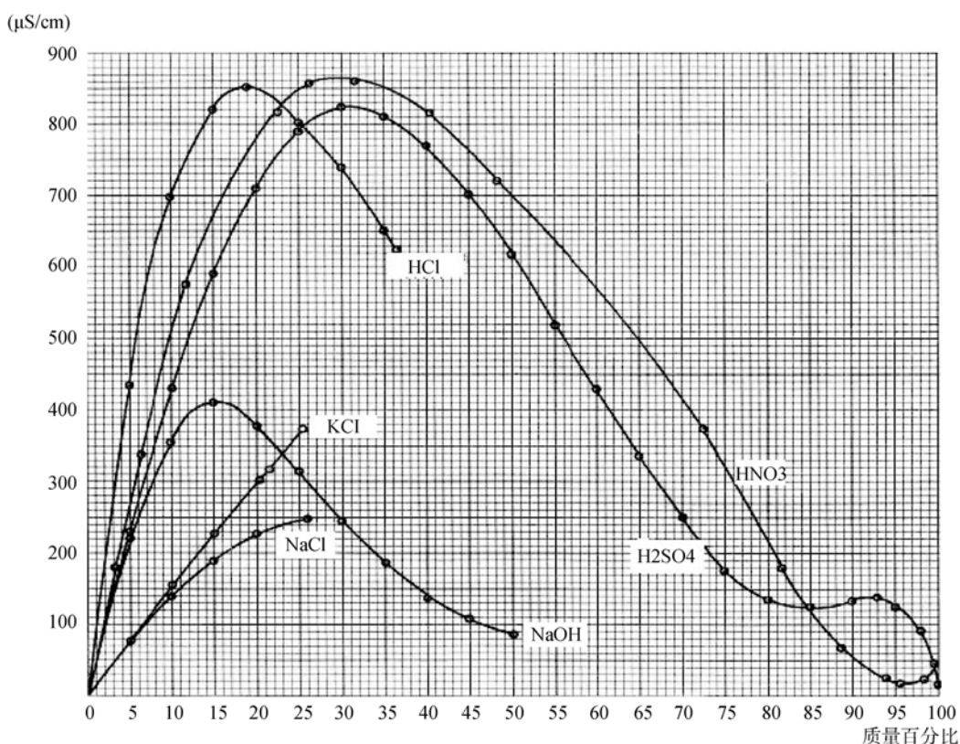
图 1 常见电解质溶液电导率与浓度对应关系(IC Technical Note., 2005 Issue 4-1)
