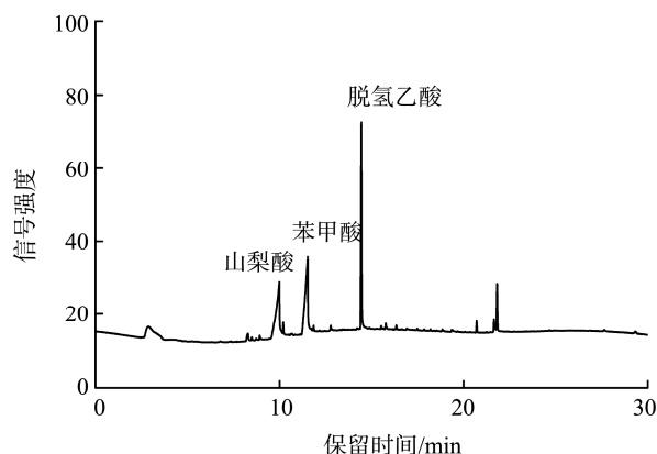
图1 山梨酸、苯甲酸和脱氢乙酸标准溶液的气相色谱图
