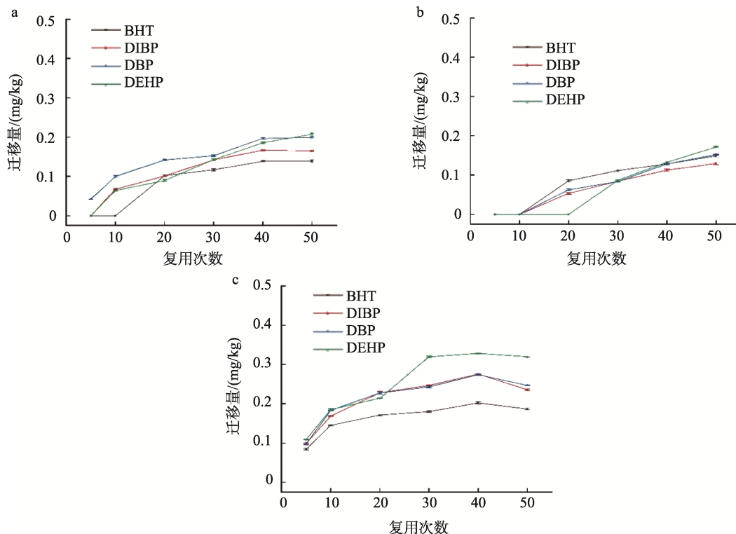
图6 热接触条件下聚丙烯餐盒复用过程向不同食品模拟物中的迁移情况(n=3)
