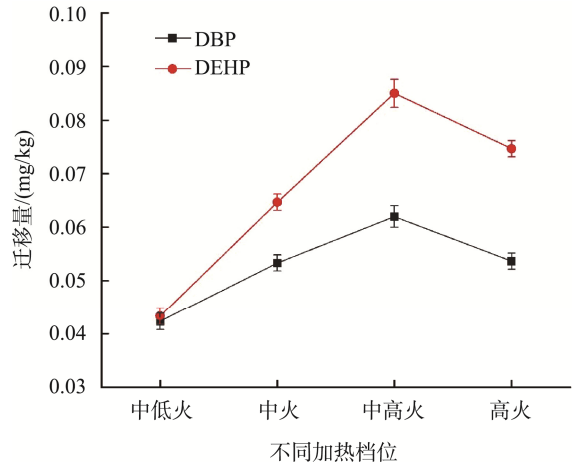
图3 微波炉不同加热档位对橄榄油中迁移量的影响(n=3)
