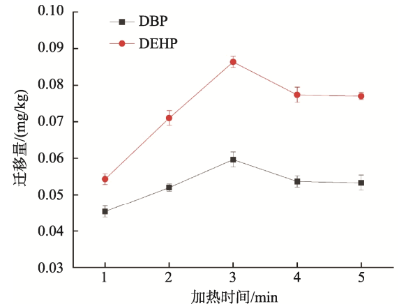
图4 微波炉不同加热时间对橄榄油中迁移量的影响(n=3)
