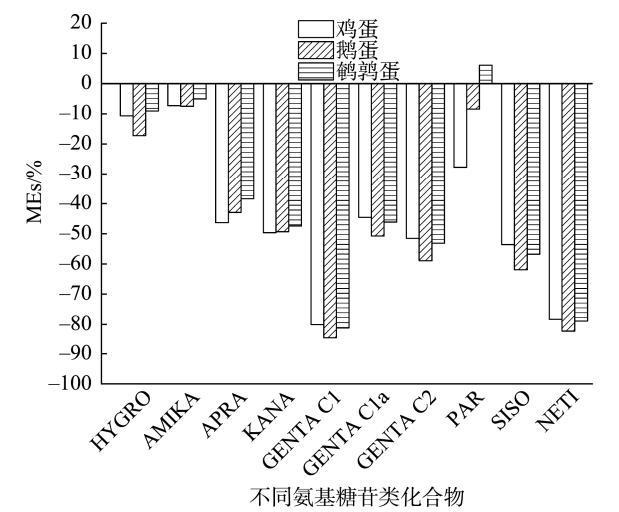
图8 10种AGs MEs的评价图 Fig.8 MEs of 10 kinds of AGs
