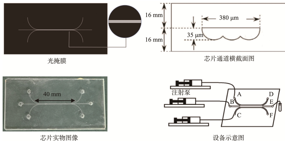
图2 微流控芯片和设备示意图
