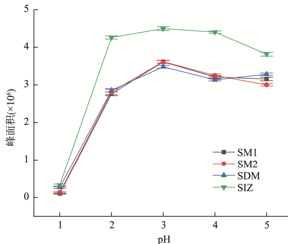
图 5 pH 对峰面积的影响( n=3 )
